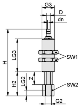
Конструктивные данные FSTIm M5-IG 6/4 A 10 IN
