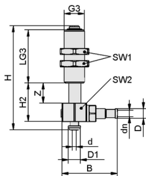
デザインデータ FSTIm N004 4/2.5 L 5 IN
