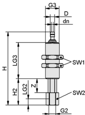
Конструктивные данные FSTIm M5-IG 6/4 A 20 VG-IN
