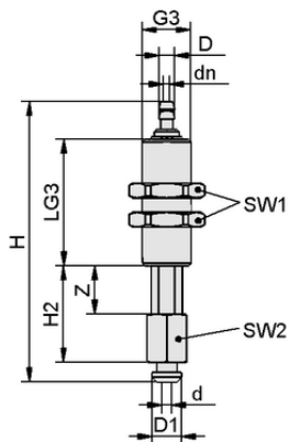
Конструктивные данные FSTIm N016 6/4 A 20 VG-IN
