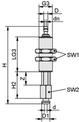
Tasarım verileri FSTIm N016 6/4 A 20 VG-IN
