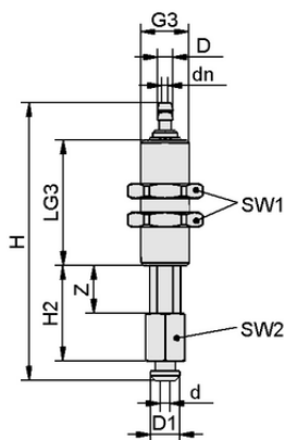
Конструктивные данные FSTIm N004 6/4 A 10 VG-IN
