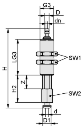
Datos de diseño FSTIm N004 6/4 A 10 VG-IN
