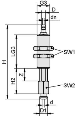
Tasarım verileri FSTIm N004 4/2.5 A 5 VG-IN
