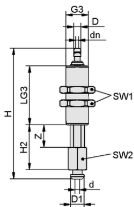
Конструктивные данные FSTIm N004 4/2.5 A 5 VG-IN
