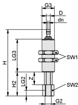
Design data FSTIm M5-IG 6/4 A 10 VG-IN
