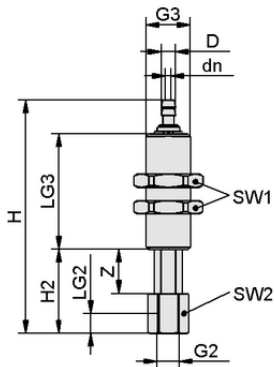
デザインデータ FSTIm M5-IG 6/4 A 10 VG-IN
