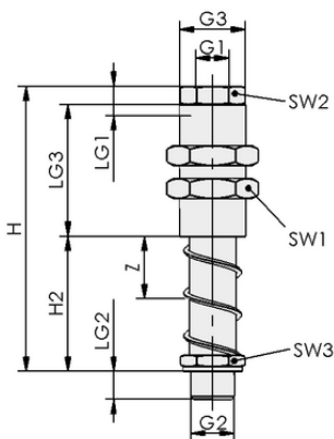
Dati di costruzione FSTE-HD G1/4-AG 90 VG
