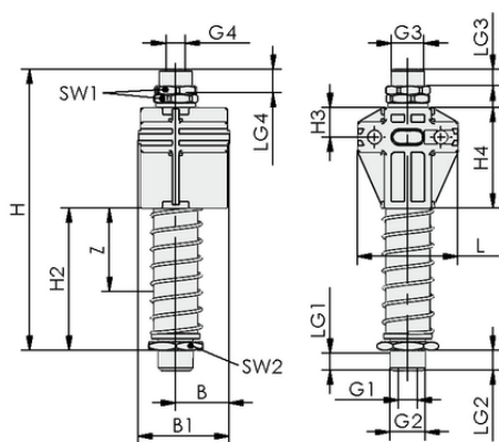
Конструктивные данные FSTF G1/2-AG 50 VG
