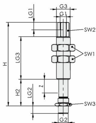
Dati di costruzione FSTI G3/8-AG G1/8-IG 50
