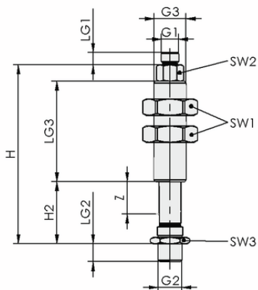
Dati di costruzione FSTI G3/8-AG G1/8-AG 50 VG
