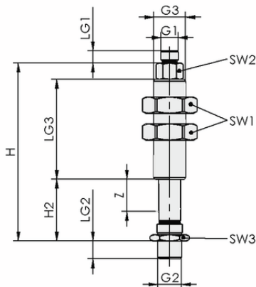
Datos de diseño FSTI G1/4-AG G1/8-AG 50 VG
