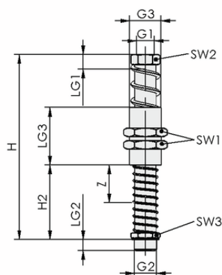
デザインデータ FSTA-HD G1/4-AG 50 VG
