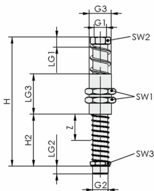
Конструктивные данные FSTA-HD G1/4-AG 50 VG
