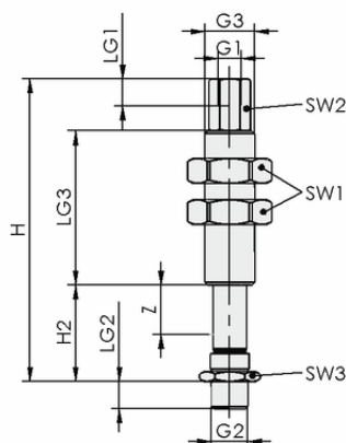
Конструктивные данные FSTI G1/4-AG G1/8-IG 25 VG
