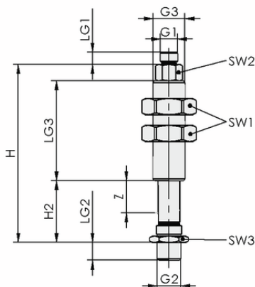
Конструктивные данные FSTI G3/8-AG G1/8-AG 10 VG
