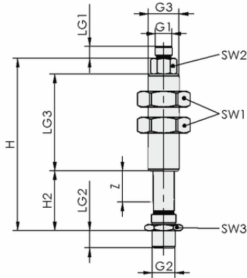
Tasarım verileri FSTI G3/8-AG G1/8-AG 25
