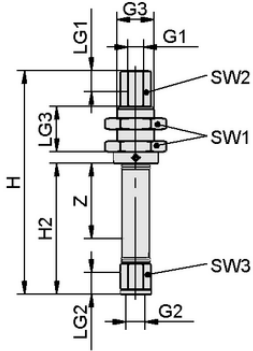
Tasarım verileri FSTE M5-IG 5 VG
