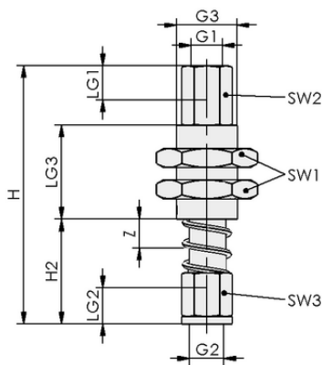
Design data FSTE M5-IG 10
