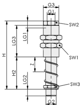
Конструктивные данные FSTE G1/8-AG 15
