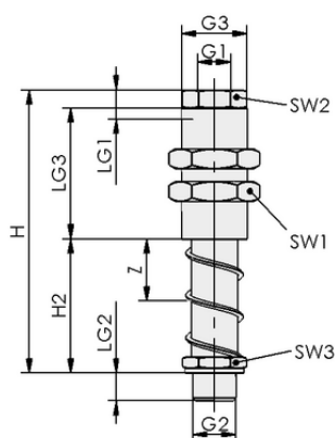
デザインデータ FSTE G1/2-AG 90
