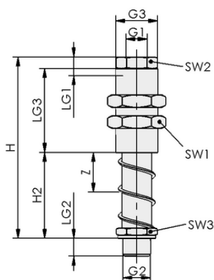
Dati di costruzione FSTE G1/2-AG 25
