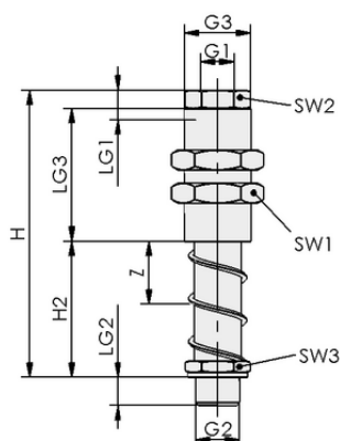
デザインデータ FSTE G1/2-AG 25
