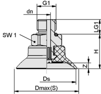
Tasarım verileri SUF 100 HT1-60 G1/8-AG
