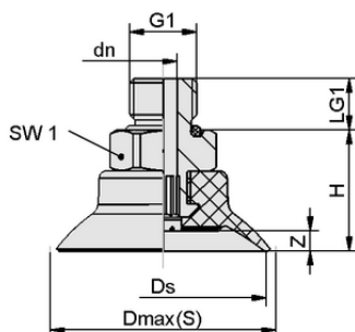
デザインデータ SUF 100 HT1-60 G1/8-AG
