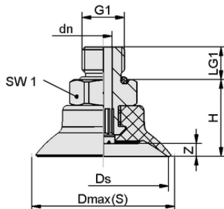
Dati di costruzione SUF 50 HT1-60 G1/8-AG
