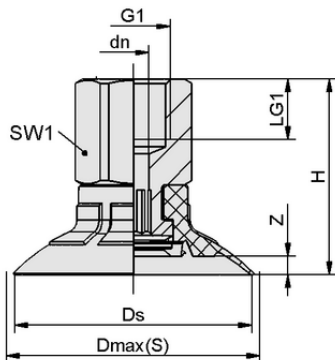
Datos de diseño SPF 30 ED-65 NPT1/8-IG
