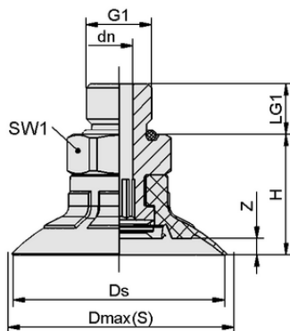
Datos de diseño SPF 30 ED-65 NPT1/8-AG
