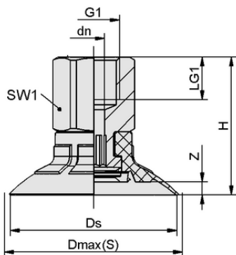
Datos de diseño SPF 25 ED-65 NPT1/8-IG
