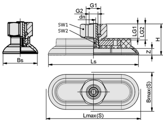
Конструктивные данные SAOG-S 80x30 NBR-60 G1/4-IG MOD
