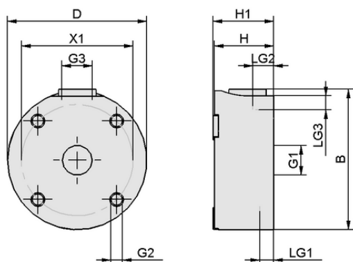
デザインデータ SBS 60 SF G1/8-IG ESD/AL
