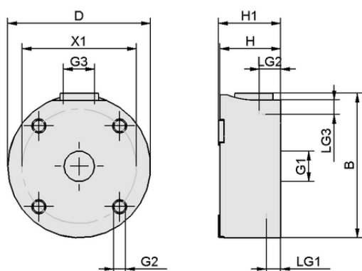
デザインデータ SBS 30 HF M5-IG ESD/AL
