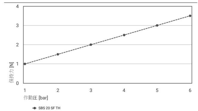
保持力
