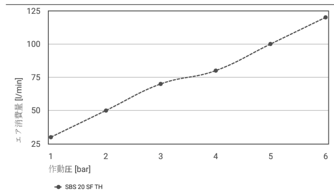
エア消費量
