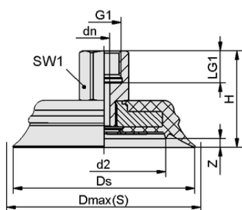
デザインデータ SHFN 50 NK-45 G1/4-IG E
