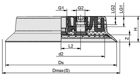
Конструктивные данные SUF 125 NBR-60 G1/4-IG
