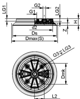
デザインデータ SUF 160 NBR-60 G1/2-IG VRS
