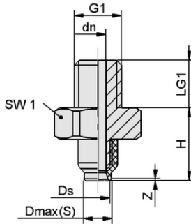
Tasarım verileri SUF 3 HT1-60 M3-AG
