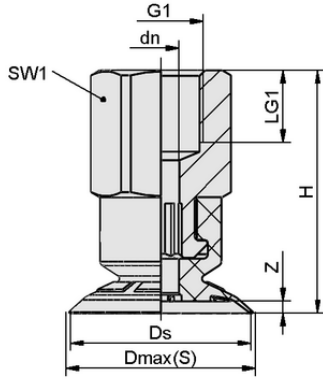
Tasarım verileri SFF 25 HT1-60 G1/8-IG
