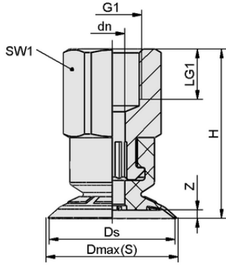
Tasarım verileri SFF 15 HT1-60 G1/8-IG
