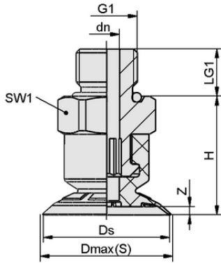
Tasarım verileri SFF 15 HT1-60 G1/8-AG
