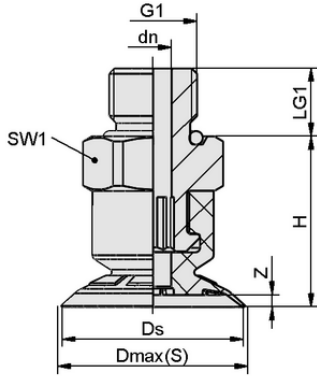
Tasarım verileri SFF 10 HT1-60 M5-AG
