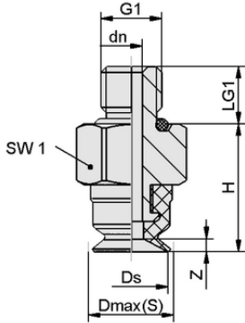
Tasarım verileri SUF 5 SI-CO-55 M5-AG
