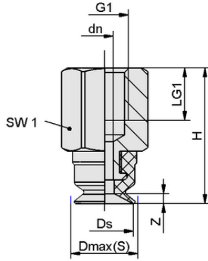
Tasarım verileri SUF 5 HT1-60 M5-IG
