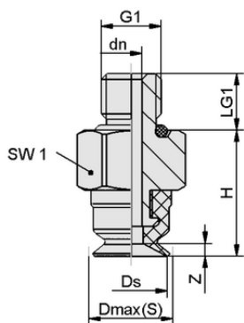
Конструктивные данные SUF 8 HT1-60 M5-AG
