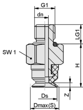
Données de construction SUF 8 SI-55 M5-AG
