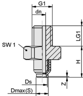
Tasarım verileri SUF 2 HT1-60 M3-AG
